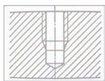
furo cego
